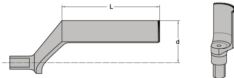
TPLO blade
